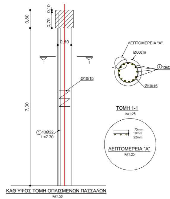
ΟΠΛΙΣΜΟΙ ΠΑΣΣΑΛΟΥ Φ600/130cm
