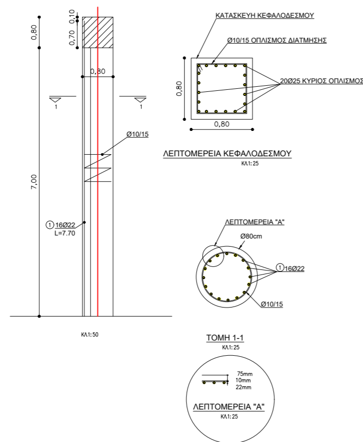
ΟΠΛΙΣΜΟΙ ΠΑΣΣΑΛΟΥ Φ800/120cm
