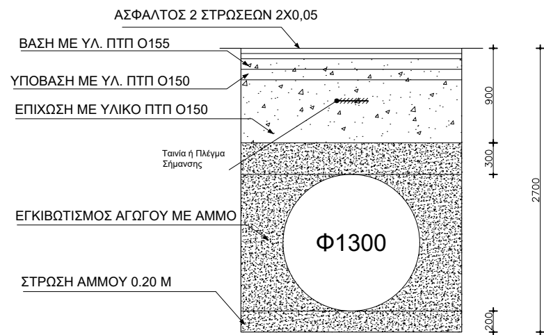
Διατομή Κλίμακα 1:50
