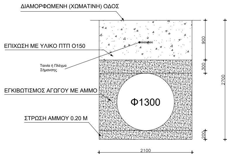
Διατομή Κλίμακα 1:50
