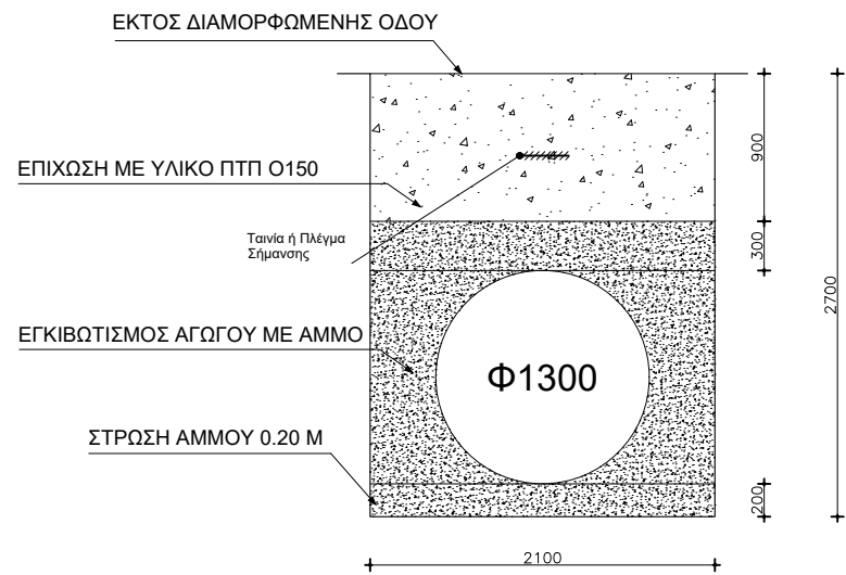
Διατομή Κλίμακα 1:50
