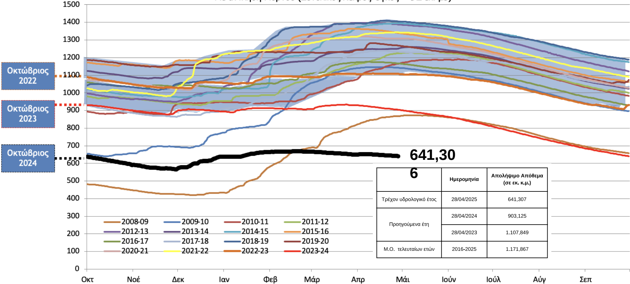
ΣΥΝΟΛΟ ΑΠΟΛΗΨΙΜΩΝ ΑΠΟΘΕΜΑΤΩΝ ΤΕΛΕΥΤΑΙΩΝ ΥΔΡΟΛΟΓΙΚΩΝ ΕΤΩΝ (σε εκ. μ3) Με άντληση Μόρνου (Συνολικός Νεκρός Όγκος = 92 εκ. μ3)
