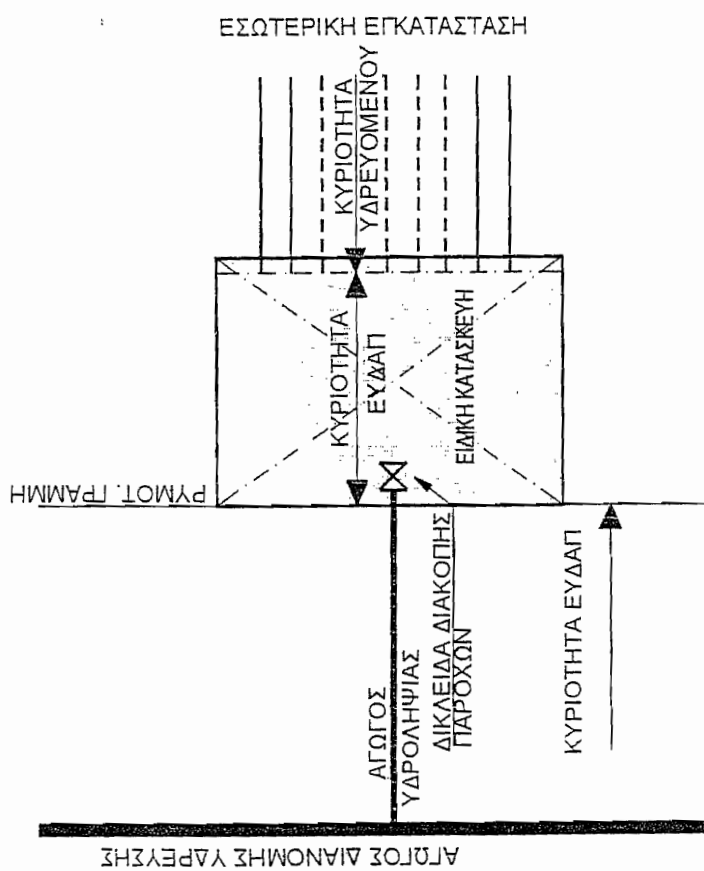
ΣΧΗΜΑΤΙΚΗ ΔΙΑΤΑΞΗ ΠΑΡΟΧΗΣ ΜΕ ΕΙΔΙΚΗ ΚΑΤΑΣΚΕΥΗ ΕΠΙ ΤΗΣ ΡΥΜΟΤΟΜΙΚΗΣ ΓΡΑΜΜΗΣ
